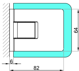
Bohrung mit Dichtung
