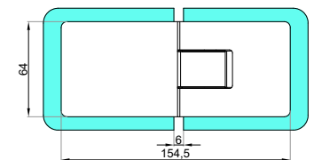
Bohrung mit Dichtung
