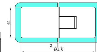
Bohrung OHNE Dichtung
